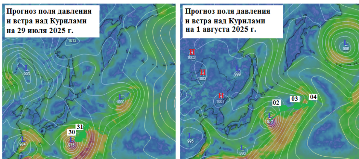
Прогностические карты приземного давления и поля ветра над Курильским районом на 29 июля и 01 августа 2025 г. (из программы Windy.map).
