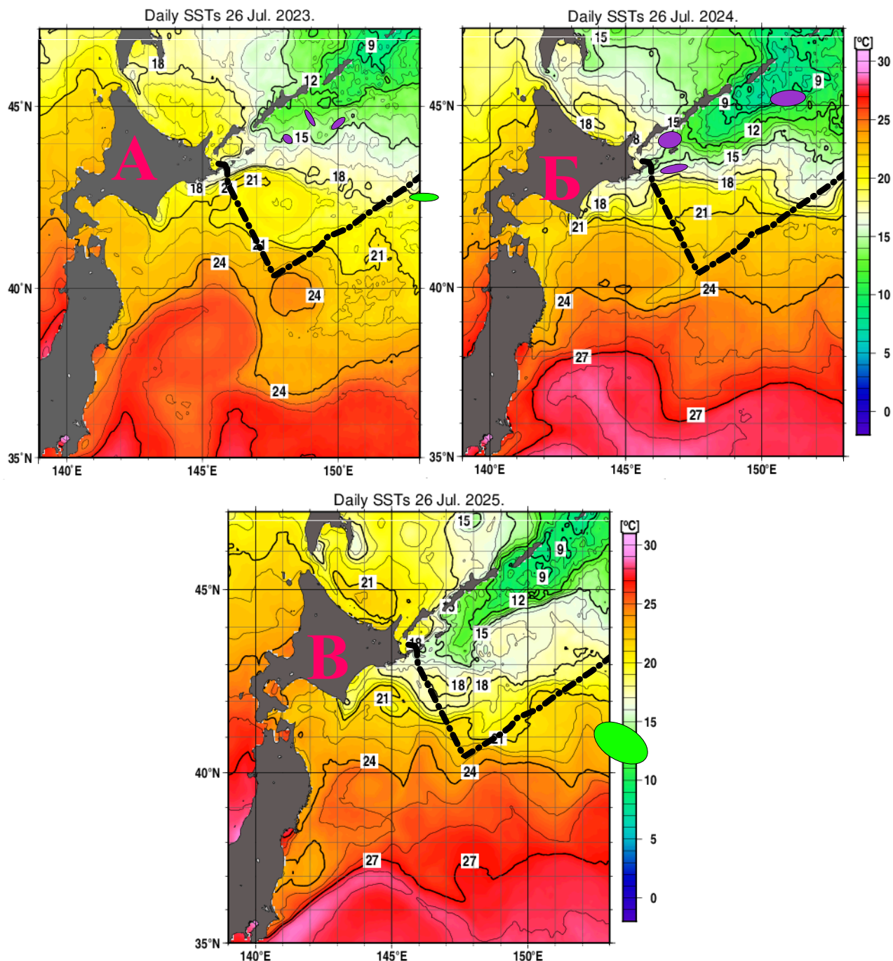
Рис. 3. Температура на поверхности океана в зоне Субарктического фронта по спутниковым данным за 26 июля 2023 (А), 2024 (Б) и 2025 (В) гг. (JMA). Показано положение изотермы 9°. Зеленым указаны районы работы иностранного флота на промысле сардины и скумбрии (в открытых водах), фиолетовым – российских судов.
