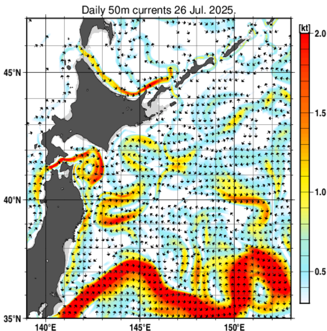
Рис. 2. Скорость и направление течений на горизонте 50 м в СЗТО за 26 июля 2025 г. (JMA)
