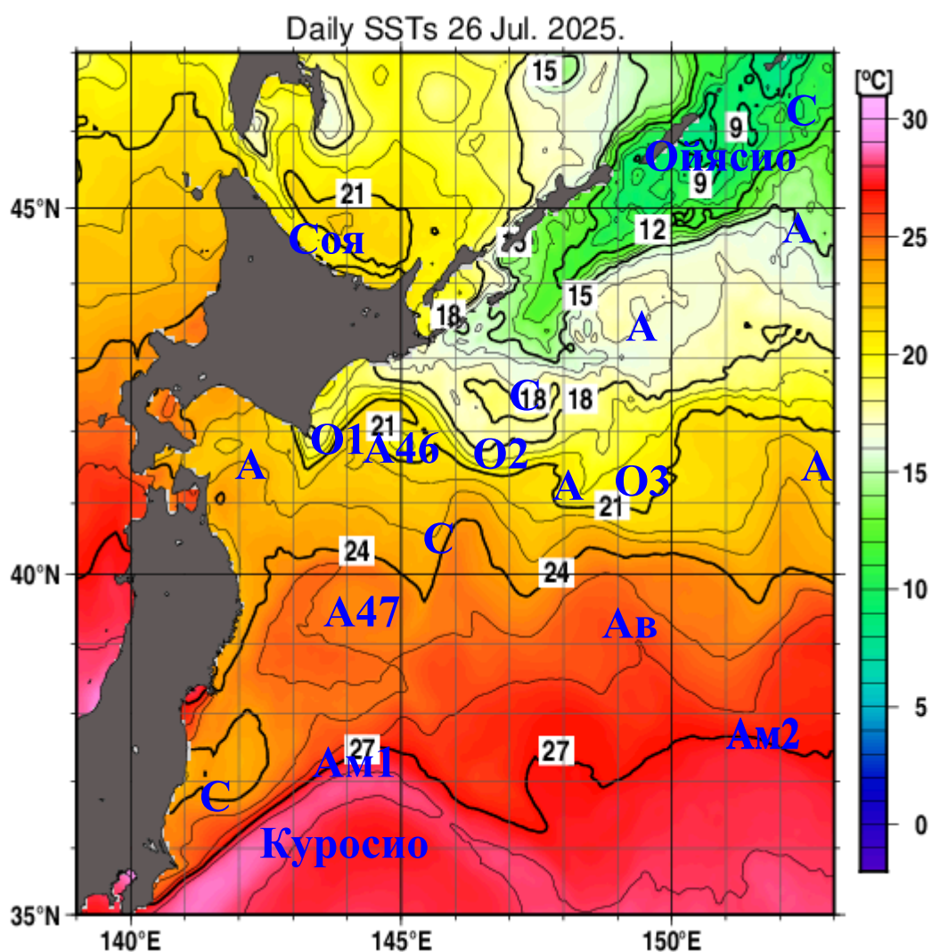
Рис. 1. Температура поверхности океана и фронтальные зоны в СЗТО по судовым и спутниковым данным за 26 июля 2025 г. (JMA)
